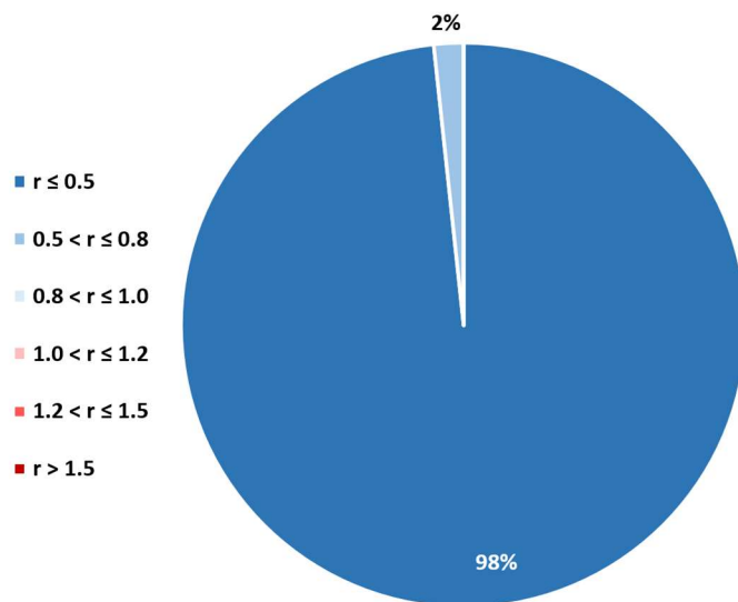
Figure 9 : fréquences des classes de ratio SumD_{2021} / SumDX en 2021
