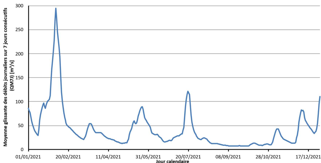
Figure 2 : la courbe du QM7J à la station d'Épinal (2021)
