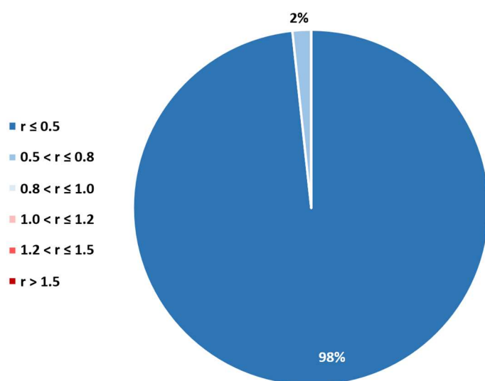
Figure 10 : fréquences des classes de ratio \text{SumVD}_{2021} / \text{SumVDX} en 2021
