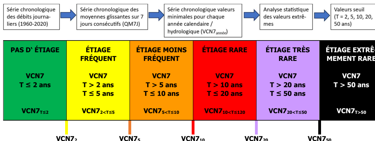
Figure 4 : la méthode de déduction de la classification des étiages à six niveaux
