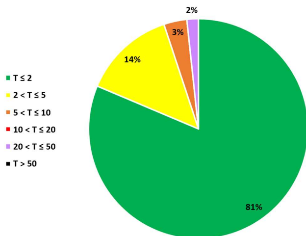
Figure 8 : fréquences des temps de retour du VCN7 (les pourcentages indiqués ont été arrondis, leur somme peut éventuellement différer des 100%)
