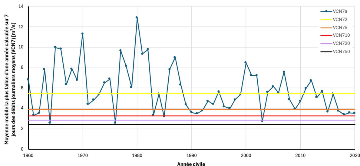
Figure 5 : la courbe du VCN7 annuel à la station d'Épinal (1960-2020) avec les valeurs seuils
