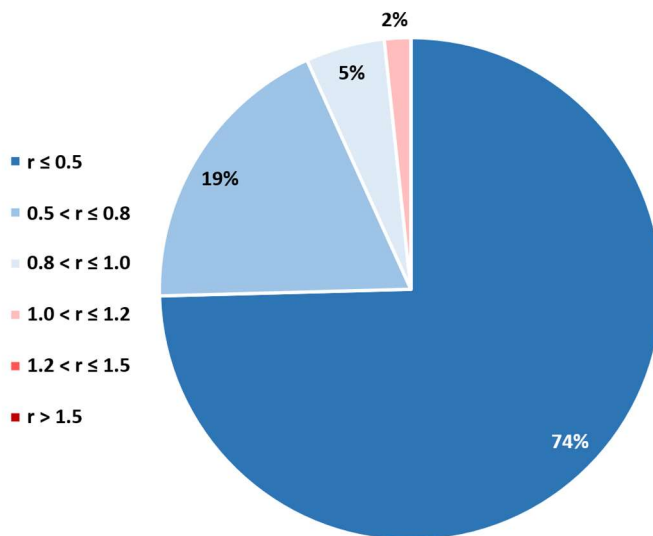
Figure 9 : fréquences des classes de ratio SumD_{2023} / SumDX en 2023
