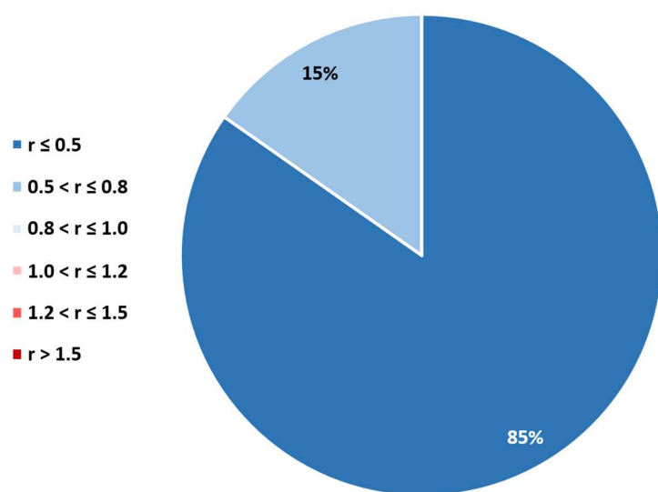
Figure 10 : fréquences des classes de ratio \text{SumVD}_{2023} / \text{SumVDX} en 2023
