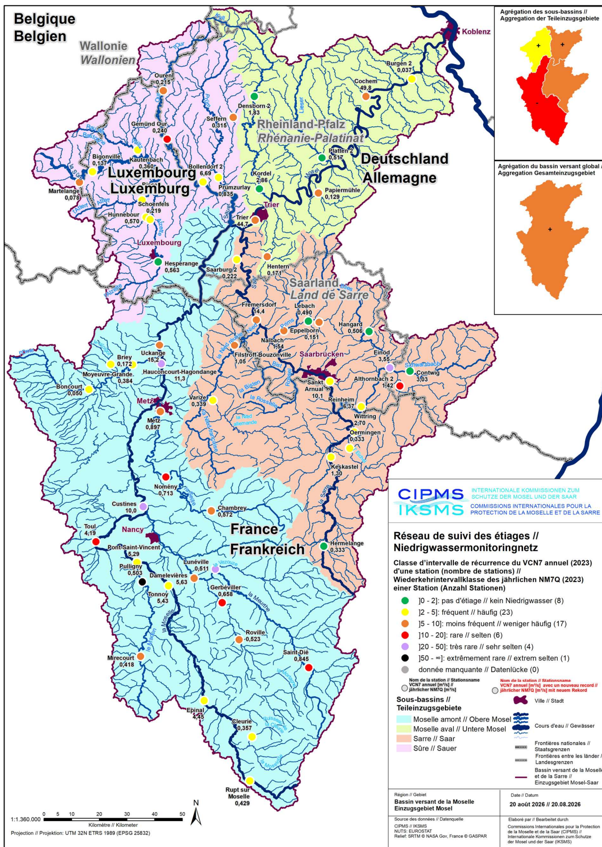
Carte 3 : VCN7 de l'année 2023 et résultats de l'agrégation à l'échelle des sous-bassins et du bassin entier
